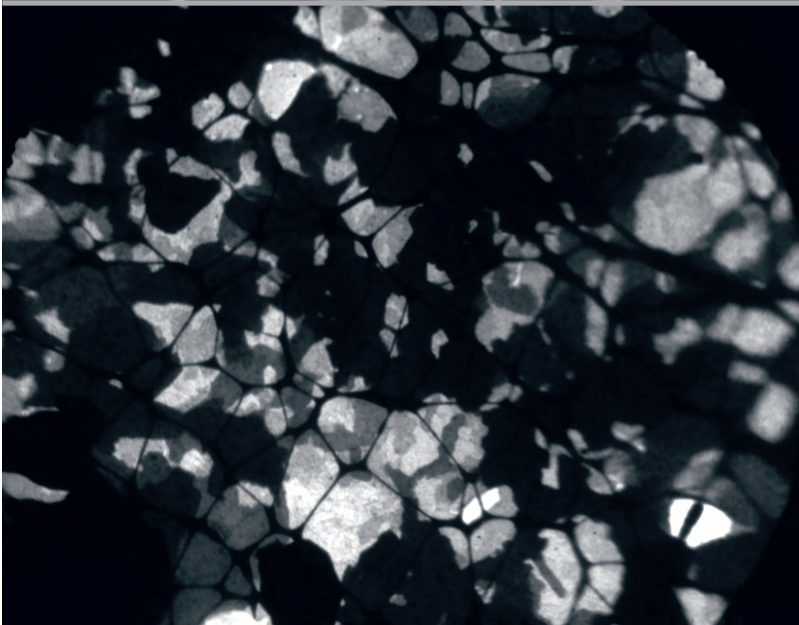
Beeld gemaakt door de elektronenmicroscopie ESCHER, ook wel: Electronic Structure CHEMical nanoimaging in Real time.
